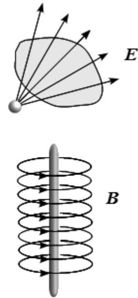
Рис. 2.2: соленоидальные поля.
