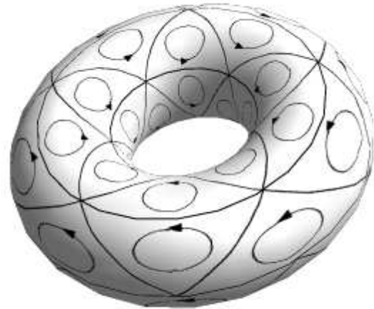
Рис. 1.8: триангуляция поверхности.
