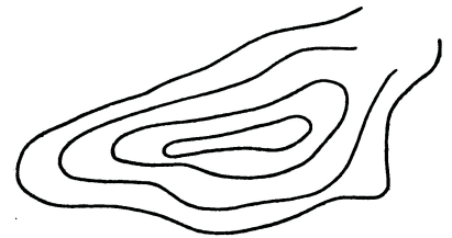
Рис. 2.1: линии уровня функции двух переменных.
