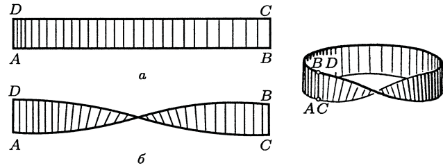
Рис. 1.6: лист Мебиуса.
