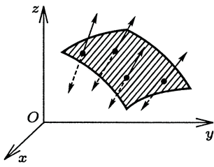
Рис. 1.5: выбор ориентации для поверхности, заданной уравнением z = f(x, y) .
