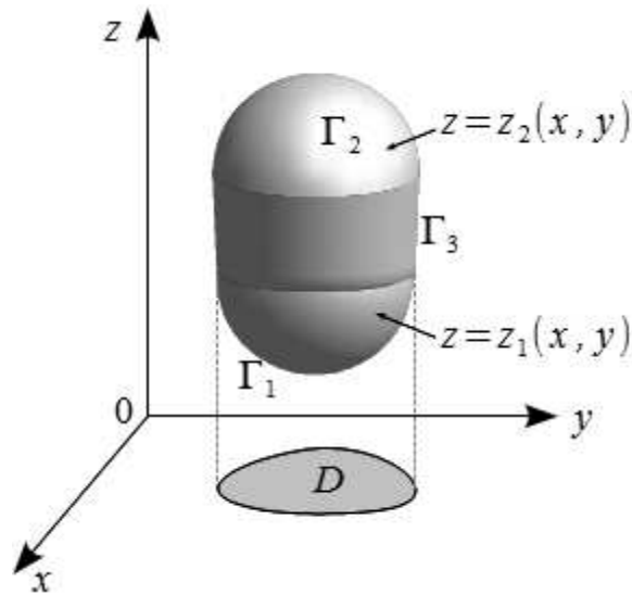
Рис. 1.9: z -цилиндрическая область.
