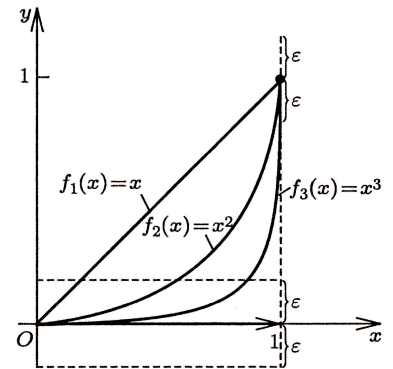
Рис. 4.1: последовательность x^k и ее предел.
