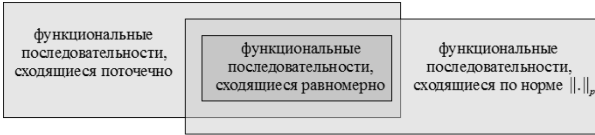
Рис. 4.5: соотношения между различными видами сходимости функциональных последовательностей: по норме \|\cdot\|_{Q[a,b]} , поточечной и равномерной.
