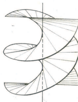
Рис. 1.2: геликоид.
