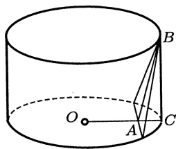
Рис. 1.3: Один слой «сапога» Шварца.
