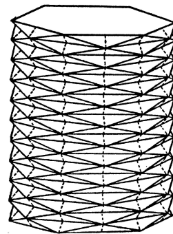
Рис. 1.4: «Сапог» Шварца.
