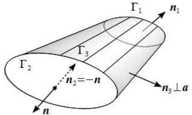
Рис. 2.3: трубка векторного поля.
