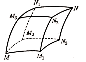
Рис. 2.4: криволинейный параллелепипед.
