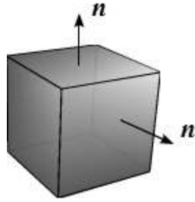
Рис. 1.7: куб.
